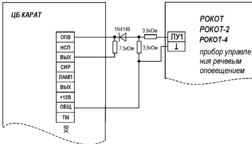
Рис. 20 Подключение прибора речевого оповещения РОКОТ, РОКОТ-2, РОКОТ-4
