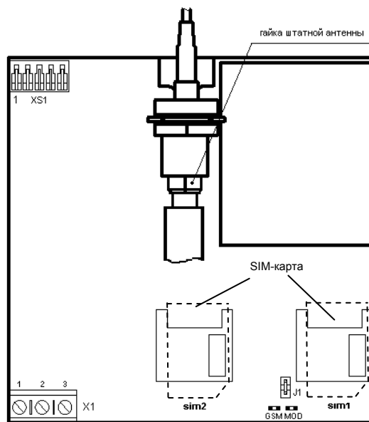
Рис. 11 Внешний вид платы универсального коммуникатора (GSM+ГТС)
