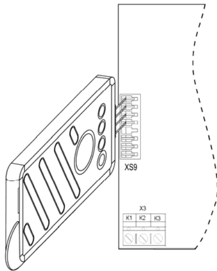
Рис. 10 Подключение USB-программатора к плате центрального блока ППКУОП «КАРАТ»
