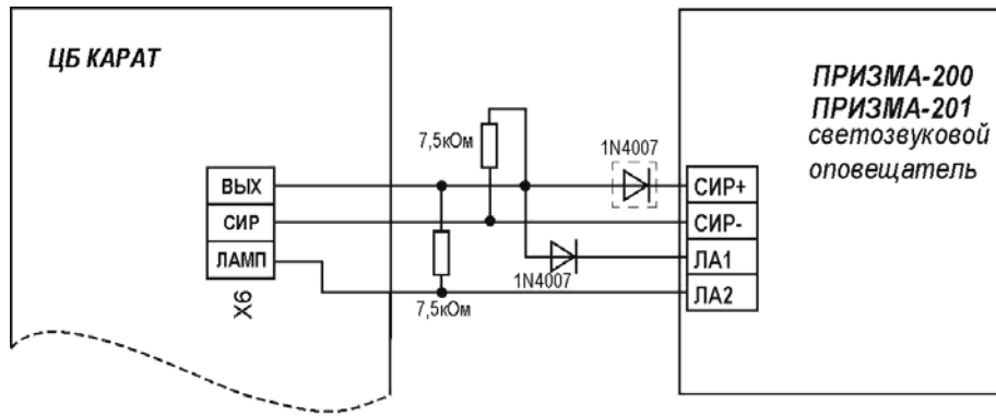
Рис. 19 Подключение светозвукового оповещателя ПРИЗМА-200 и ПРИЗМА-201
