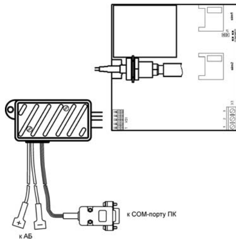
Рис. 14 Подключение адаптера программатора к универсальному коммуникатору
