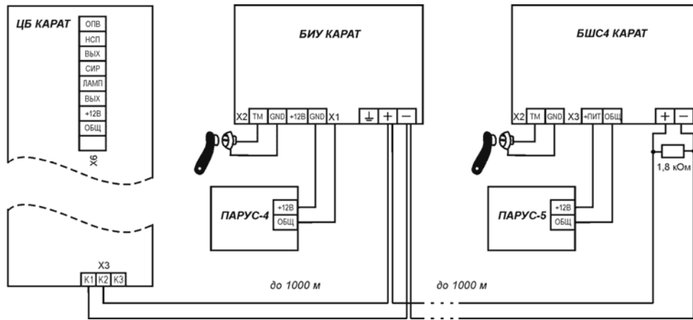
Рис. 6 Схема соединения БИУ, БШС4 и ЦБ
