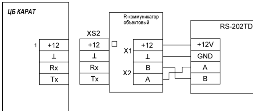
Рис. 17 Схема соединения прибора с R-коммуникатора и передатчиком
