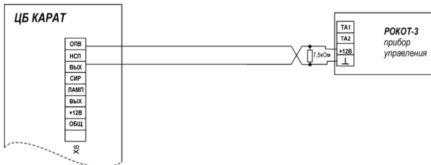
Рис. 21 Подключение прибора речевого оповещения РОКОТ-3
